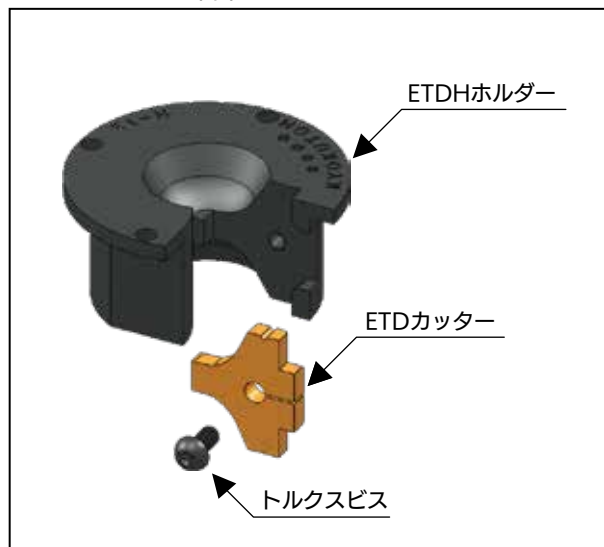
カッターホルダー詳細図
